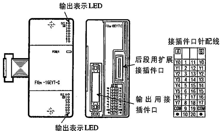
FX 2 N-16EYT-C 晶体管输出 16 点
