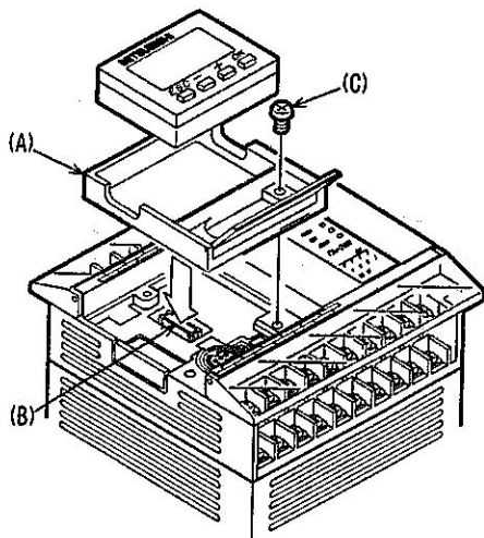
《FX 1N -5DM 的安装》
