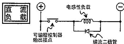
《输出回路的构成》
