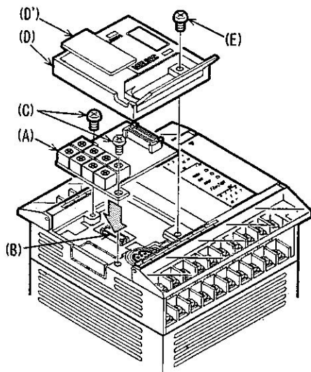
《功能扩展板的安装》
