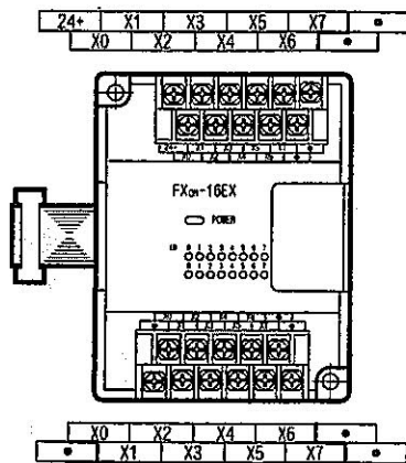
FX0N-16EX 直流输入 16 点
