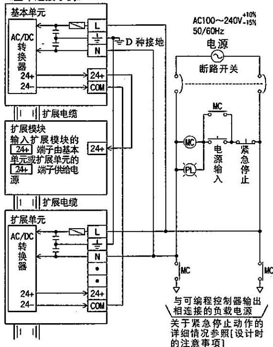
《基本连接示例》
