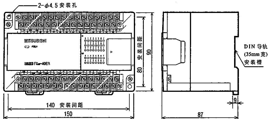
FX ON 系列扩展单元
