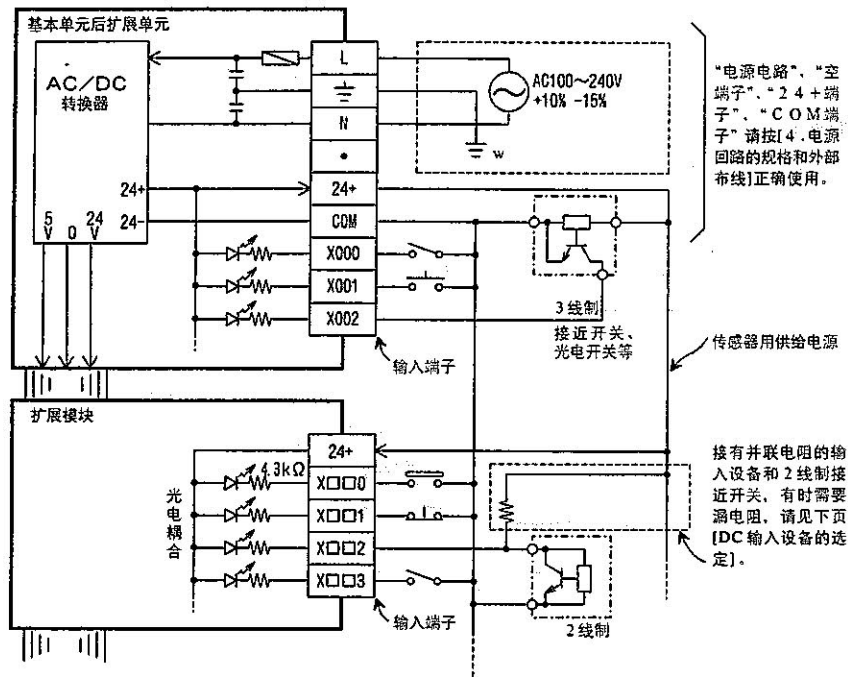
《输入连接例》
