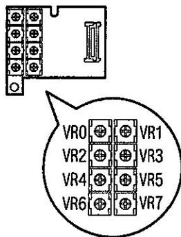
电位器放大图
