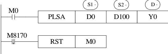
《16 位指令形式》
