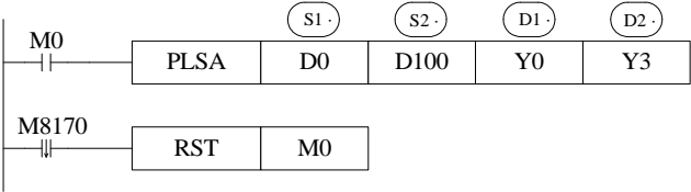
《16 位指令形式》
