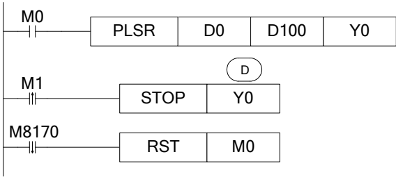
《16 位指令形式》
