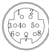
Mini Din 8 芯插座（孔）
