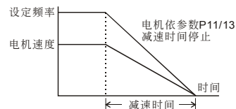
图一：减速刹车
