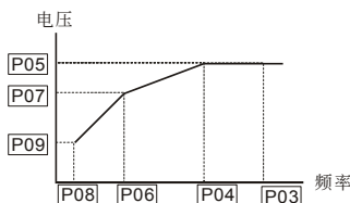
图二: 任意V/F曲线设定
