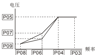
图三: 特殊V/F曲线设定
