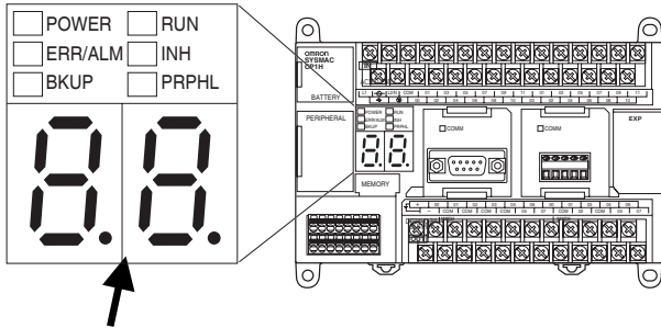
7 节 LED×2 位
