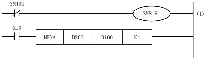
(1): 16位转换模式
