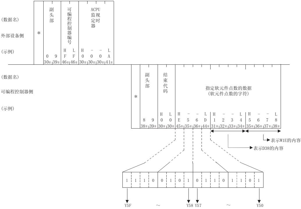
(b) 通过 ASCII 代码进行通信时
