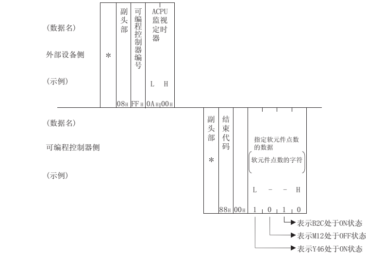
(b) 通过 ASCII 代码进行通信时
