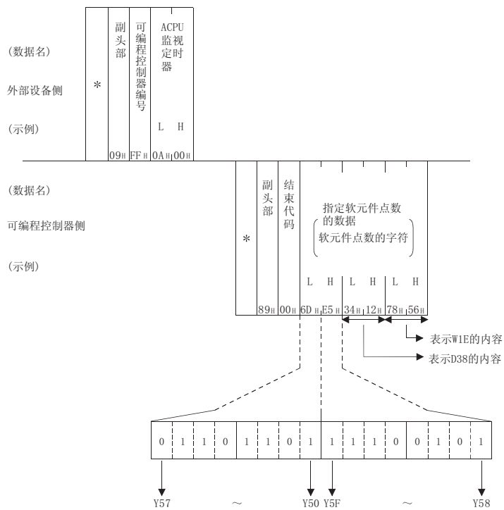
(a) 通过二进制代码进行通信时
