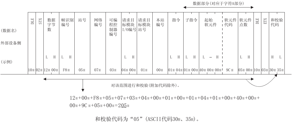
(示例 2) 以 QnA 兼容 4C 帧格式 5 进行数据读取的情况下
