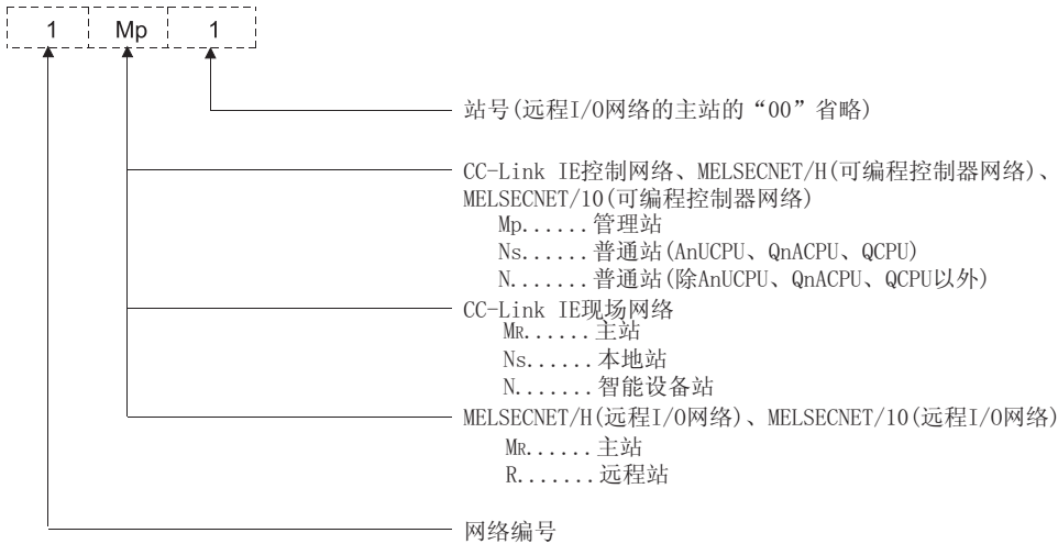
(a) CC-Link IE 控制网络、MELSECNET/H(可编程控制器网络)、MELSECNET/10(可编程控制器网络)的情况下 • 二级系统时
