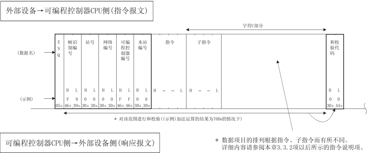
(b) 外部设备对本站可编程控制器 CPU 进行数据写入的情况下
