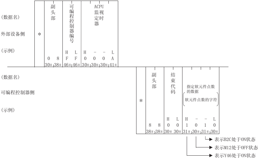
(b) 通过 ASCII 代码进行通信时
