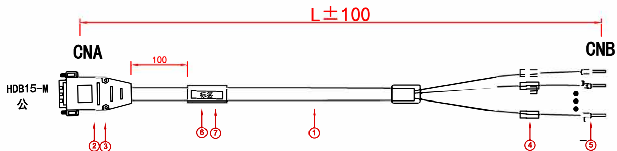
松下配线图
