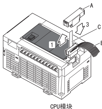
CPU模块
