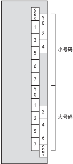
FX5-16EYR/ES FX5-16EYT/ES
