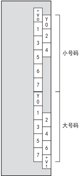
FX5-16EYT/ESS
