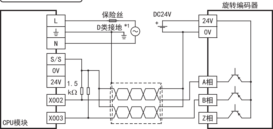
源型接线时
