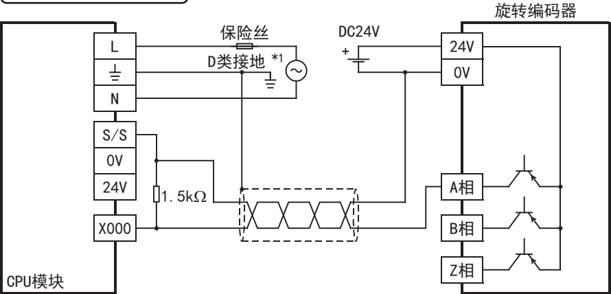
源型接线时
