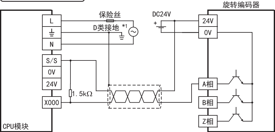
漏型接线时
