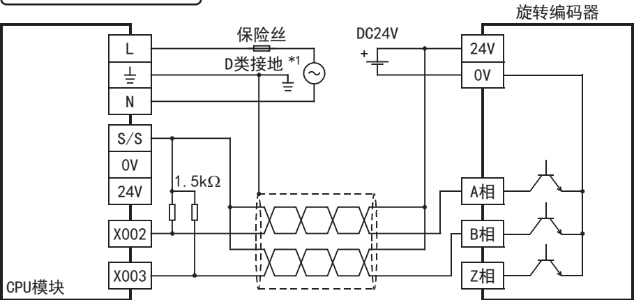
漏型接线时
