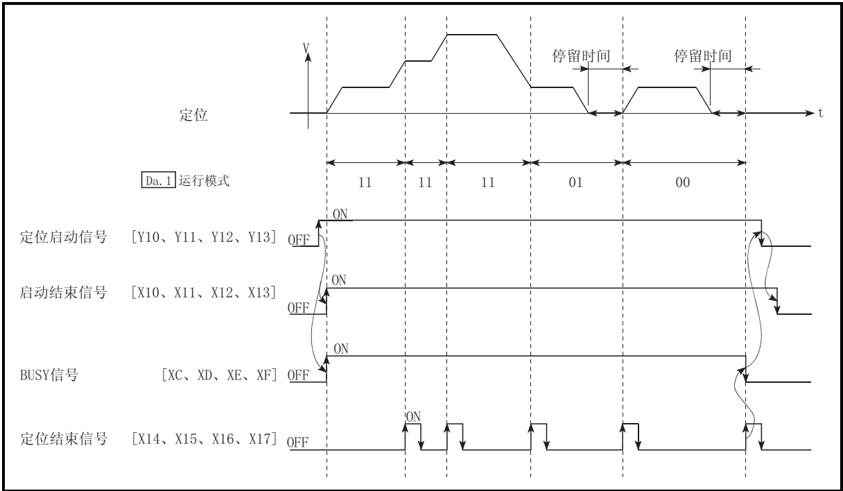
图 9.5 前置速度切换模式时的动作
