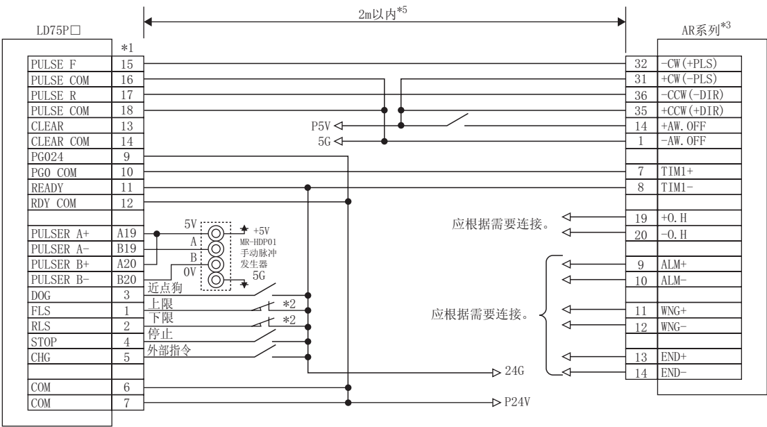
■LD75P□与 AR 系列的连接示例(开集电极) *4
