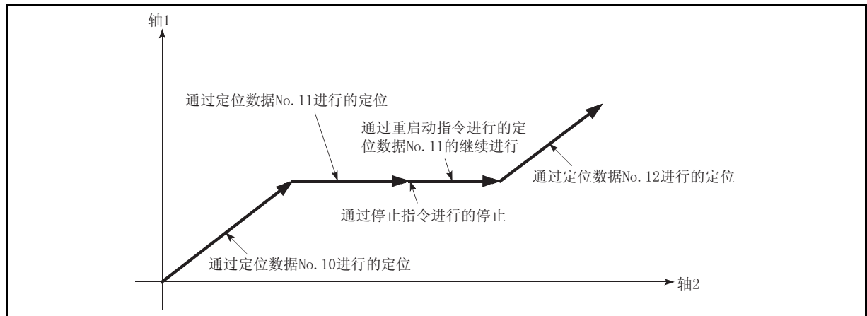
图 6.13 重启动的动作
