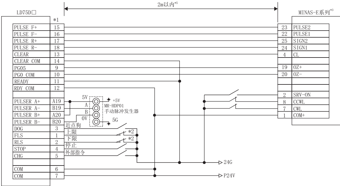
■LD75D□与 MINAS-E 系列的连接示例(差动驱动) *4
