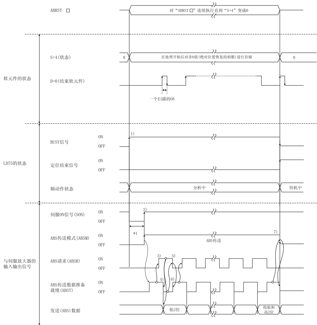
图 12.36 绝对位置检测时的信号状态
