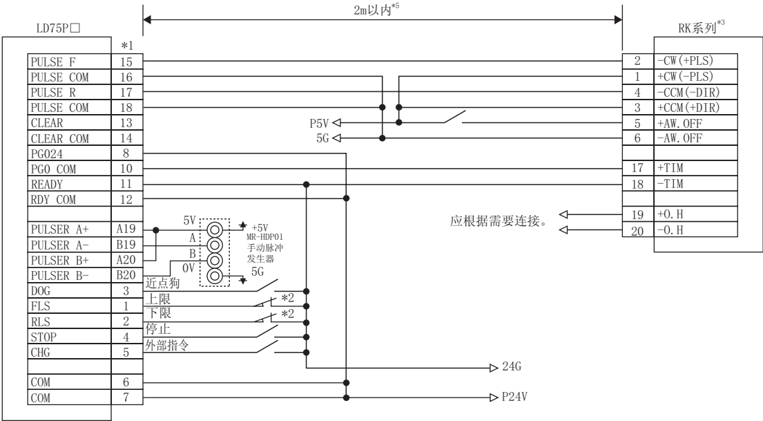
■LD75P□与 RK 系列的连接示例(开集电极) *4
