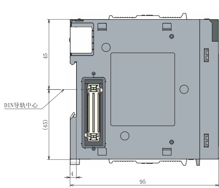
[1] LD75P1
