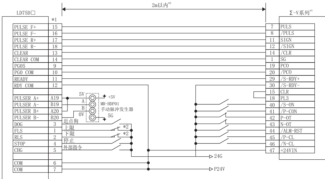
■LD75D□与 \Sigma -V 系列的连接示例(差动驱动)*4
