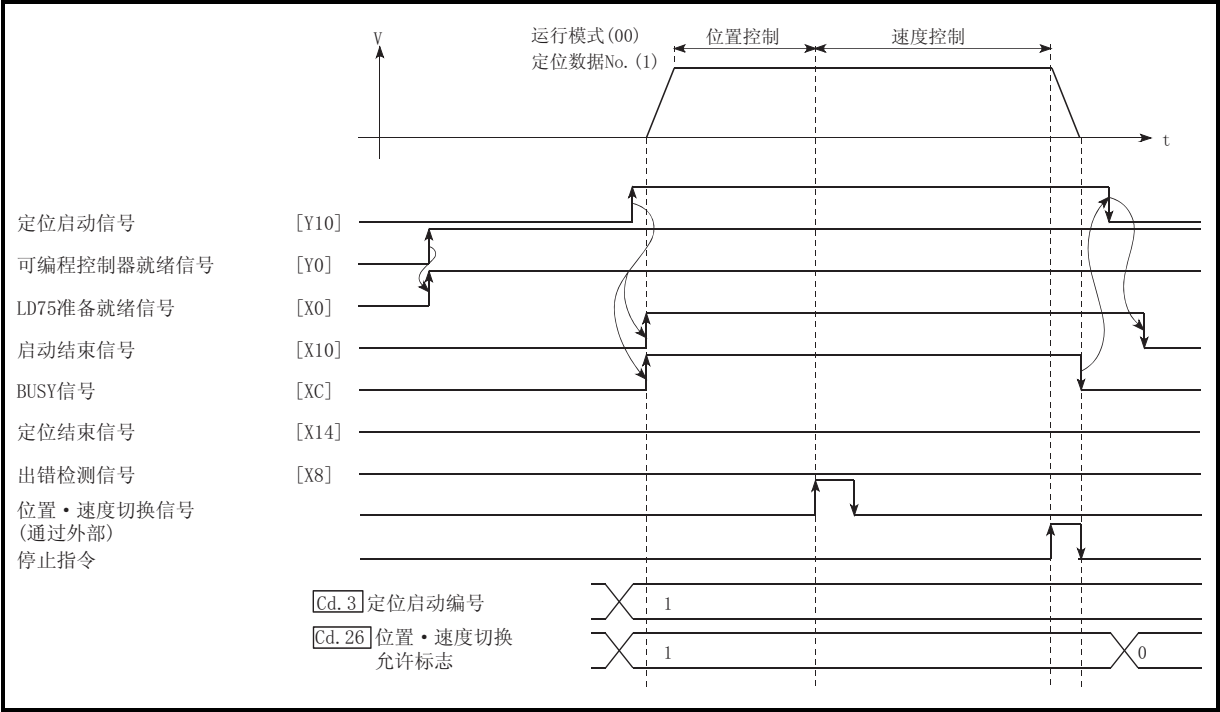
图 6.8 位置 · 速度切换控制的启动用时序图
