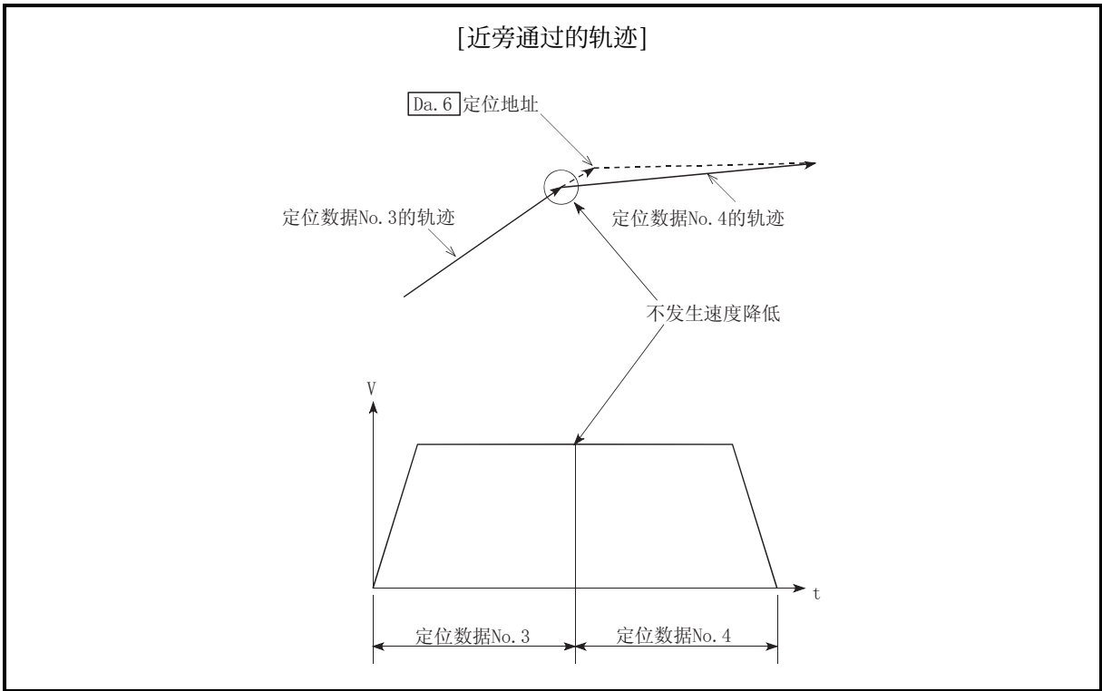
图 12.11 连续轨迹控制时的轨迹
