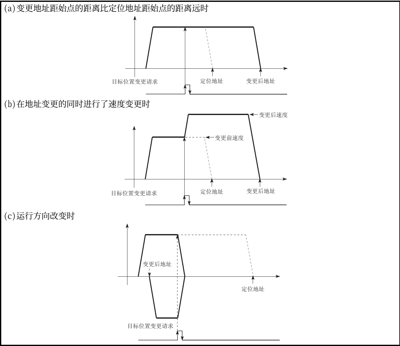
图 12.31 目标位置变更的动作
