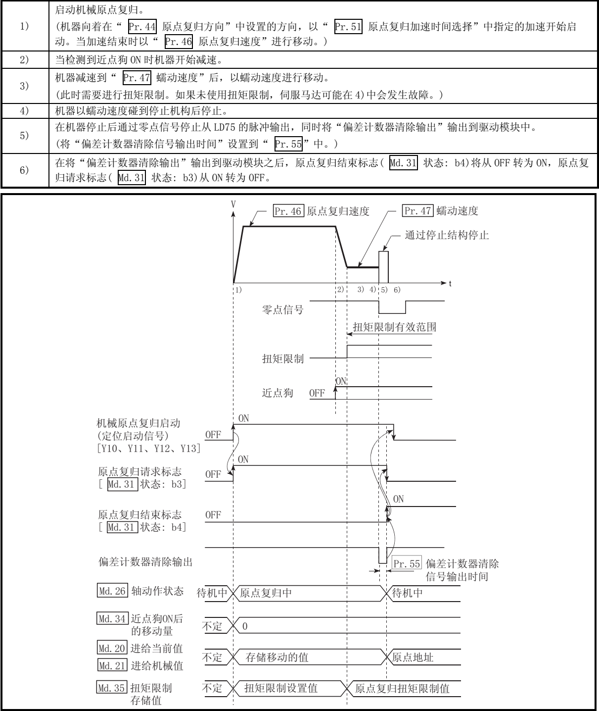
图 8.7 停止机构停止式 2) 的机械原点复归
