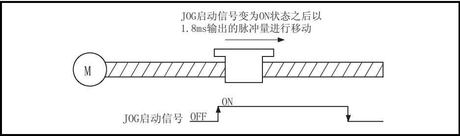
图 11.2 微动运行
