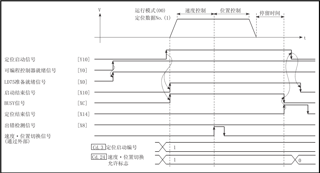
图 6.7 速度 · 位置切换控制的启动用时序图
