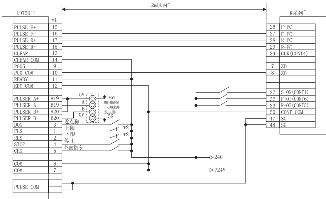
■LD75D□与 R 系列的连接示例(差动驱动)*4
