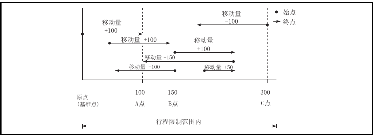
图 9.7 递增方式的定位
