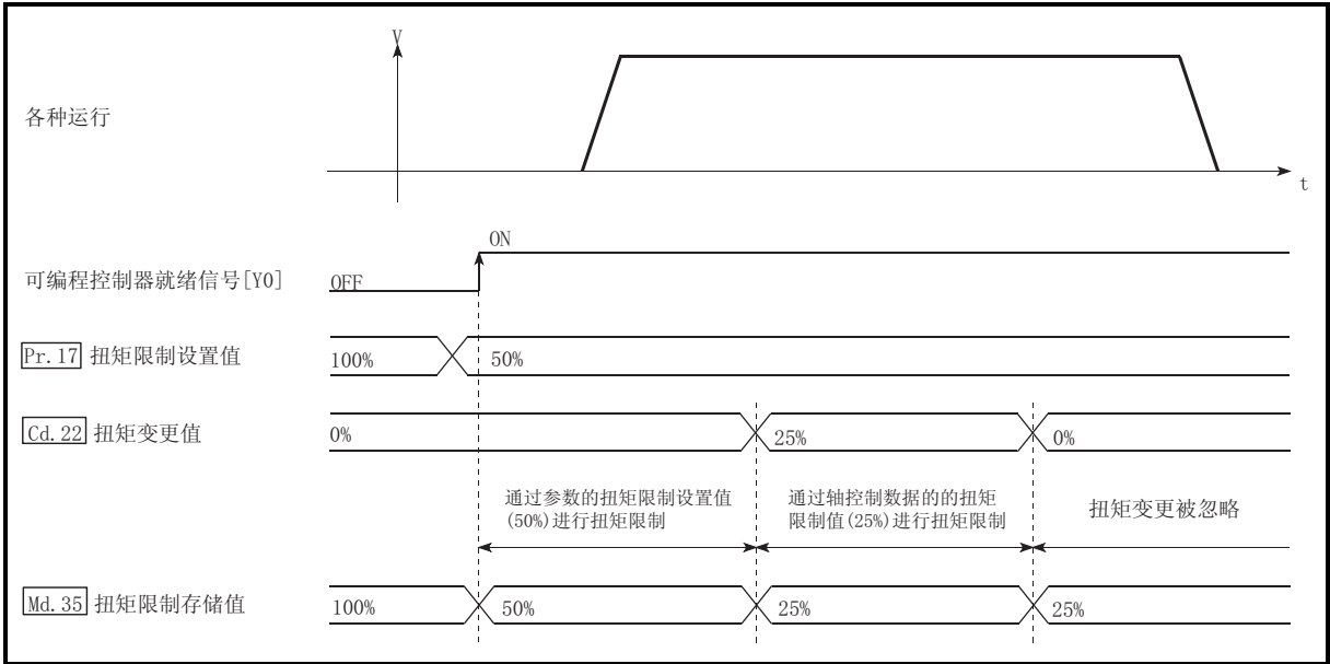
图 12.30 扭矩变更的动作
