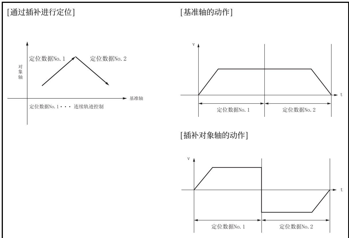
图 12.12 连续轨迹控制中移动方向改变时的轨迹及各轴的输出速度
