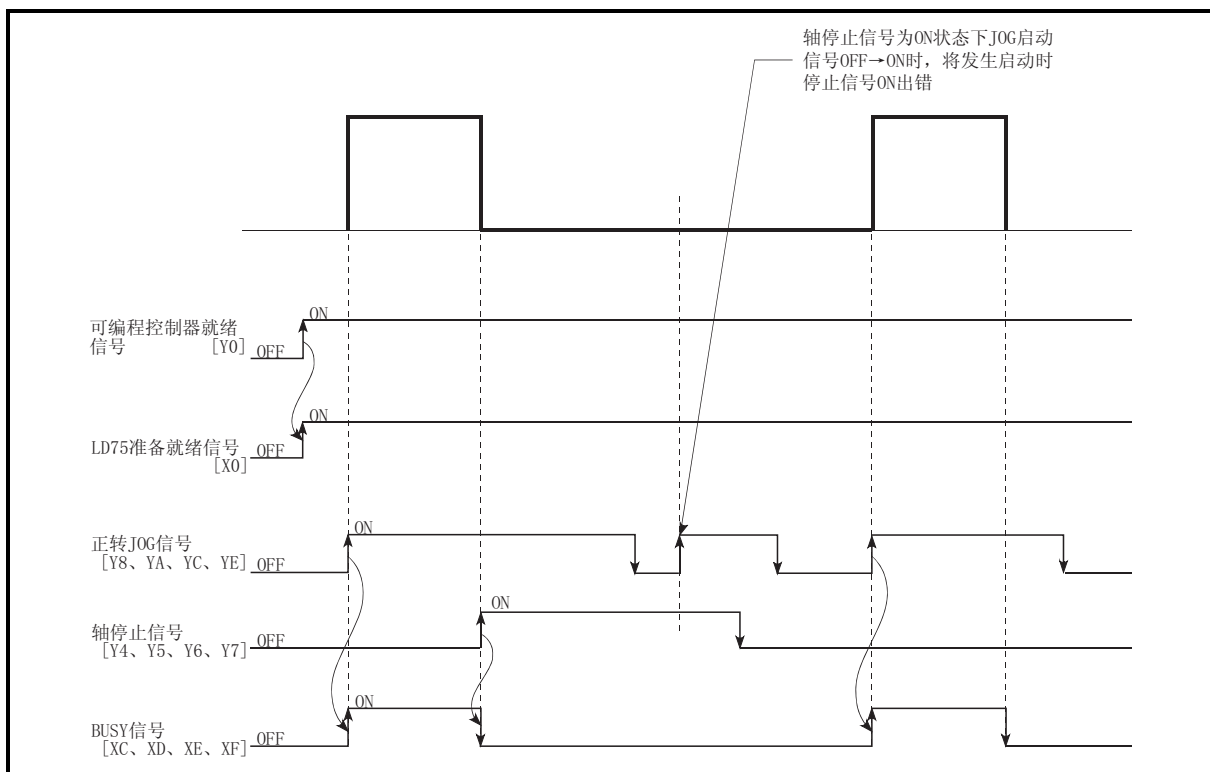
图 11.14 停止信号处于 ON 状态下进行了微动运行时的动作
