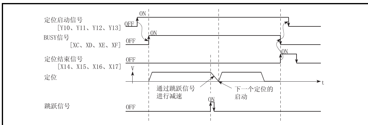
图 12.39 定位控制中输入了跳转信号时的动作
