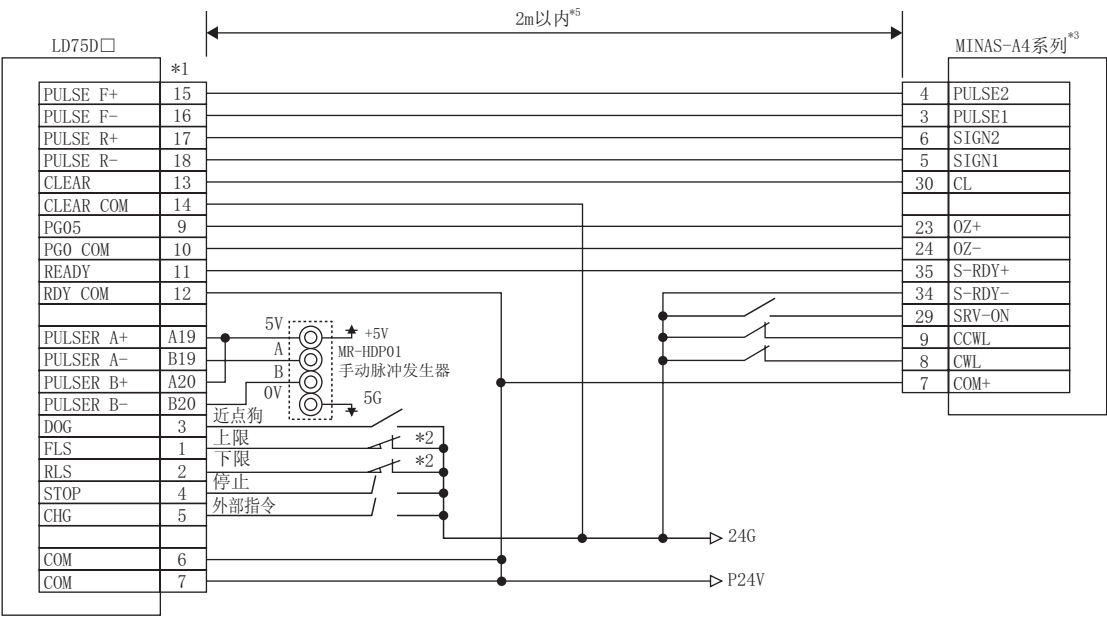
■LD75D□与 MINAS-A4 系列的连接示例(差动驱动)*4
