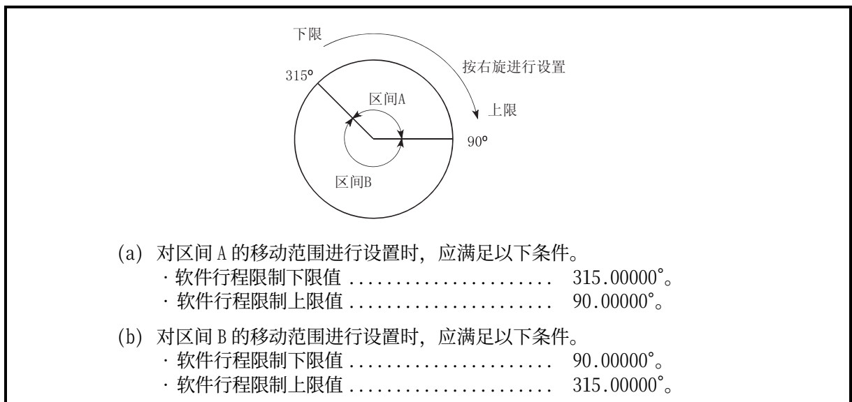
图 12.18 控制单位为“degree”时的软件行程限制
